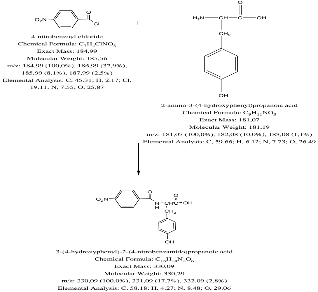
Şekil 3.2. N-p-nitrobenzoil-L-tirozin yapısı
