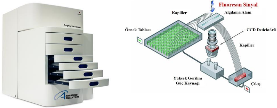
Şekil 3.5. Fragman analizörü ve çalışma sistemine ait görseller
