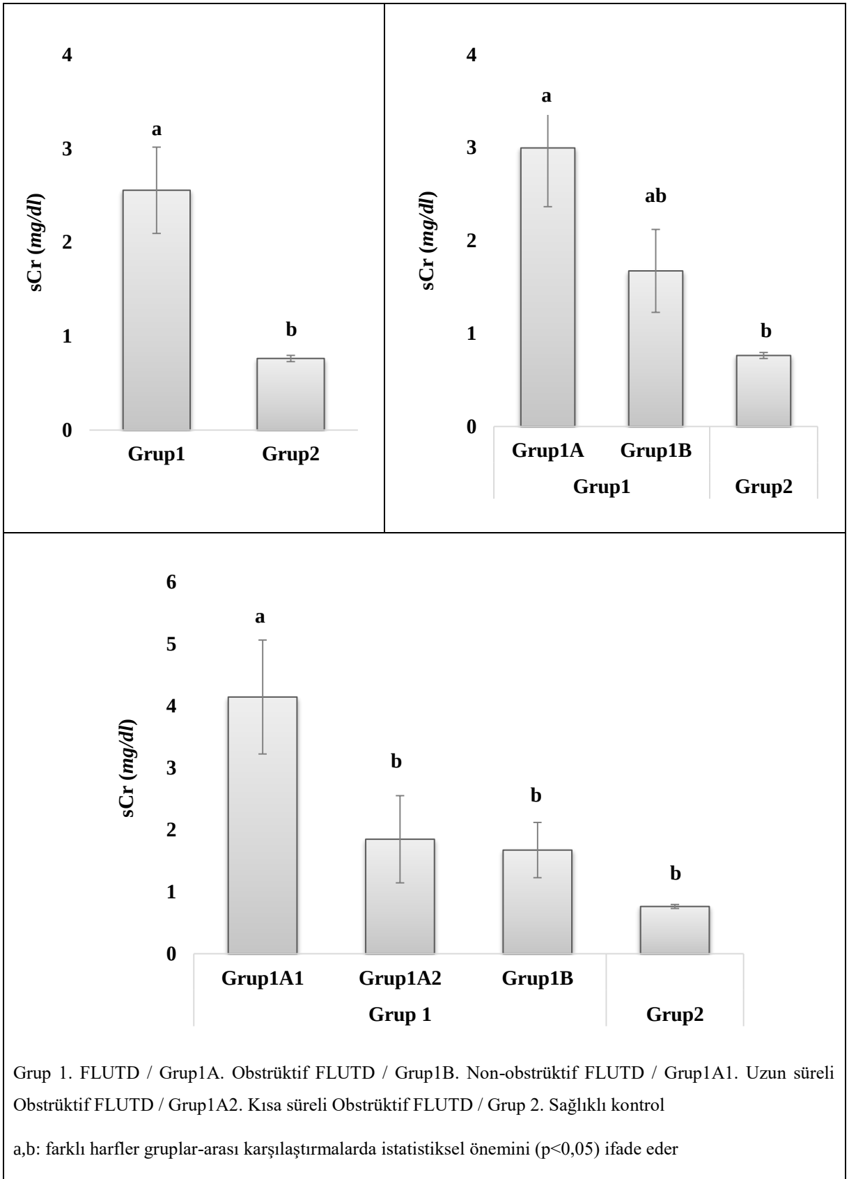
Şekil 5. Çalışma gruplarının serum kreatin (sCr) konsantrasyonları ve gruplar-arası istatistiksel değerlendirmeleri.
