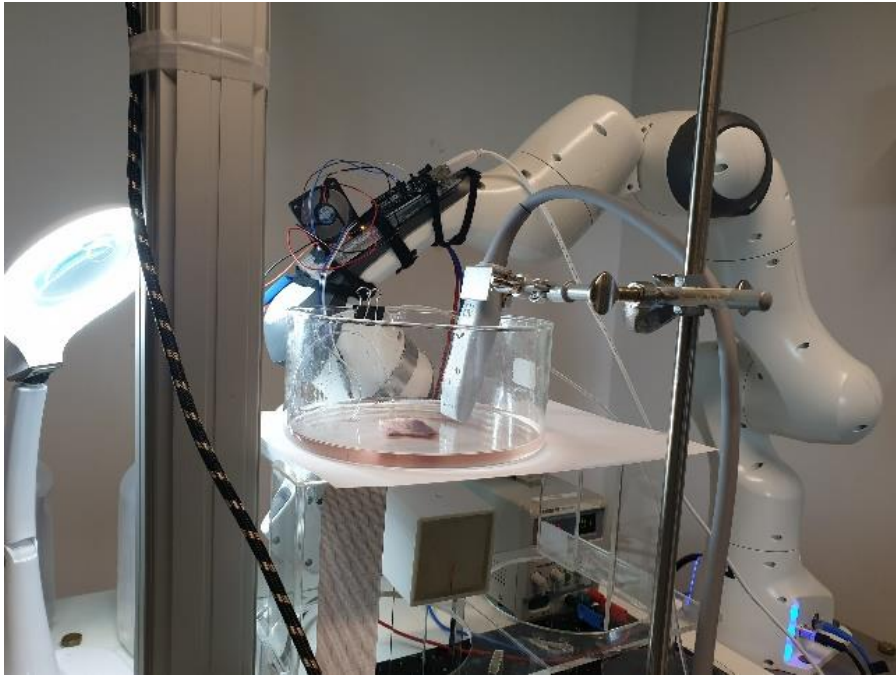
Resim 13. Mikrorobotun, robotik kola baęlı sabit mıknatıs (5x5 cm) ile domuzdan elde edilmi  arter l menleri i inde sonografi e lięinde hareket ettirilmesi.
