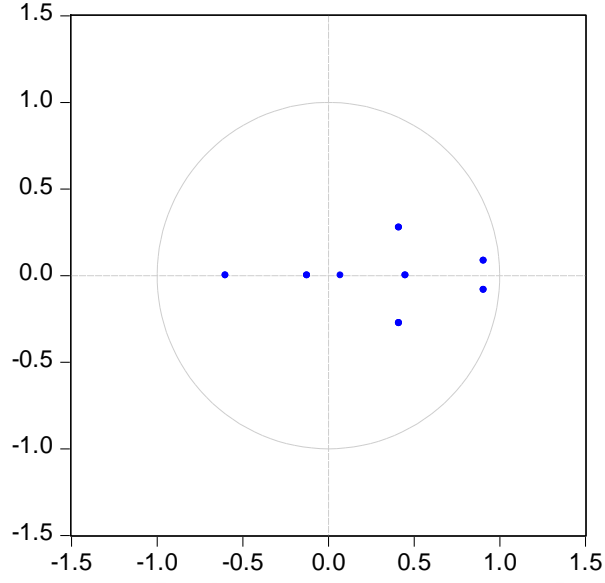
Grafik 3.2.: İkinci Modele Ait AR Karakteristik Polinomunun Ters Kökleri
