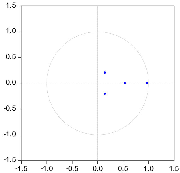
Grafik 3.1.: Birinci Modele Ait AR Karakteristik Polinomunun Ters Kökleri
