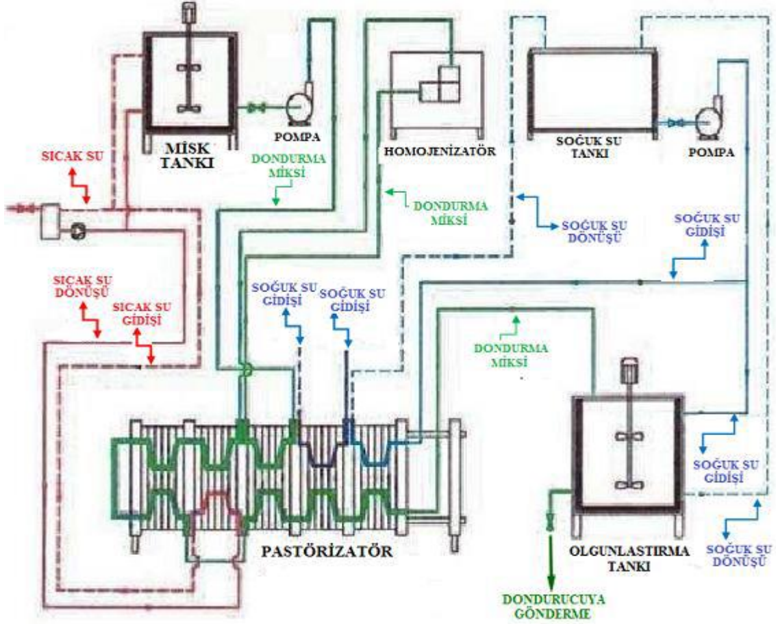
Şekil 5. Dondurma işlenmesinin şematik görünümü (Web_8, 2016)
