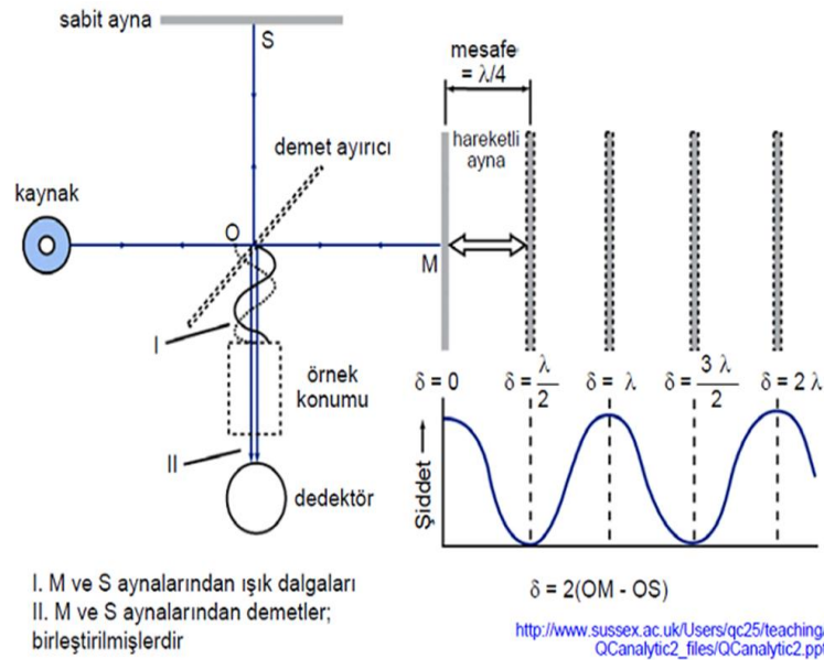
Şekil 10. Michelson interferometresi
